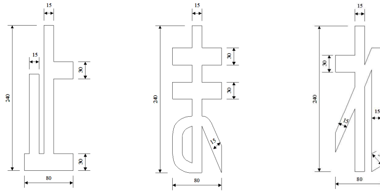
図例(1) 標準寸法図
