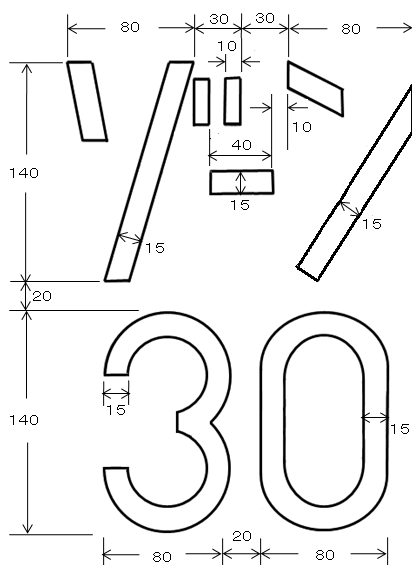
図例(1) 標準寸法図
