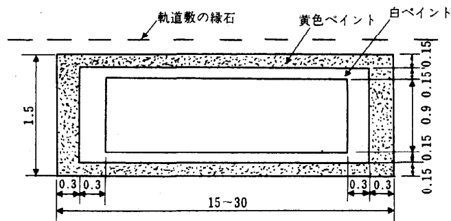
図例(2) 設置例
